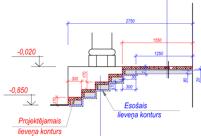
Griezums 4 - 4 M 1:50
