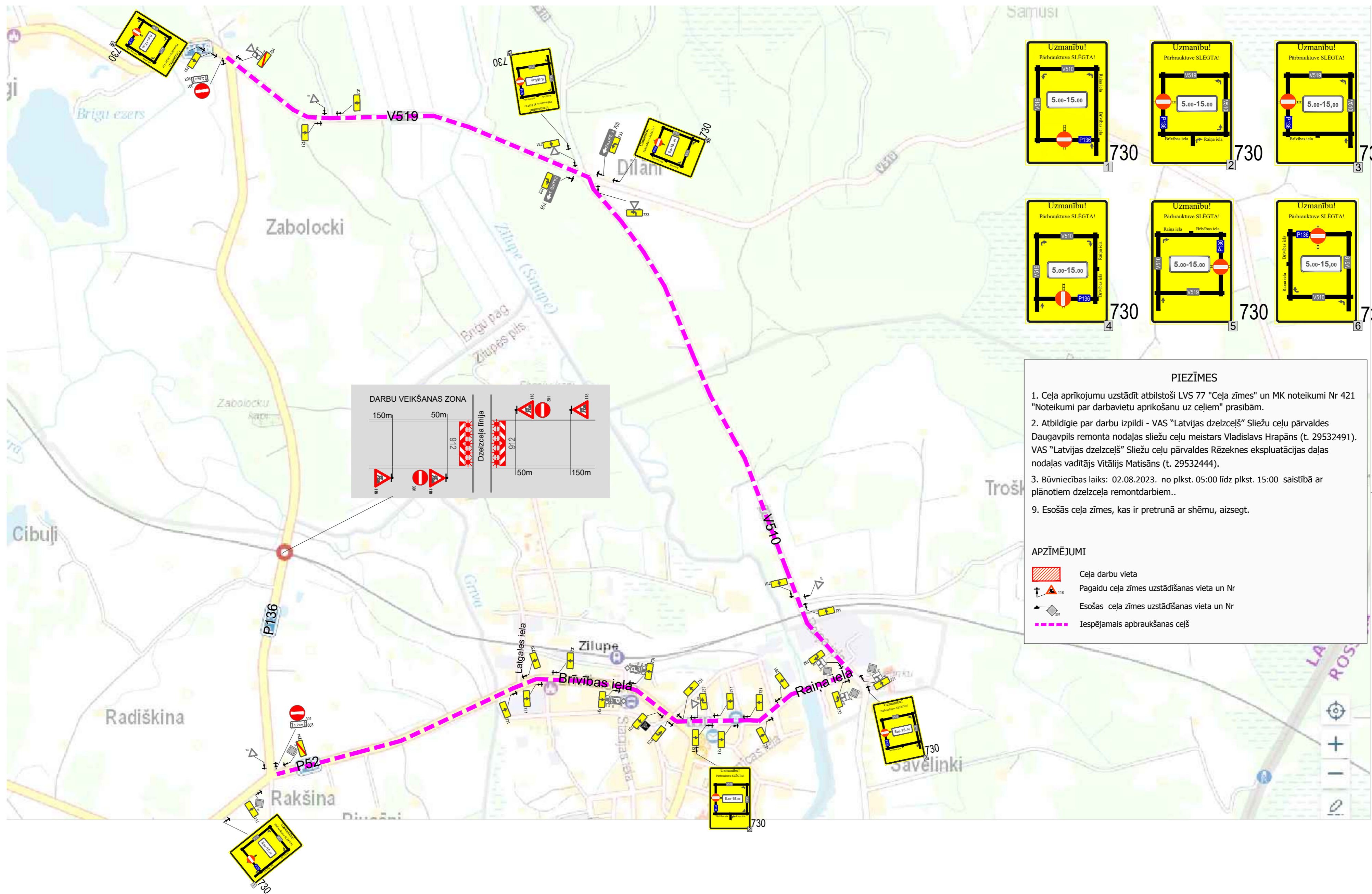
Shēma Nr.1
