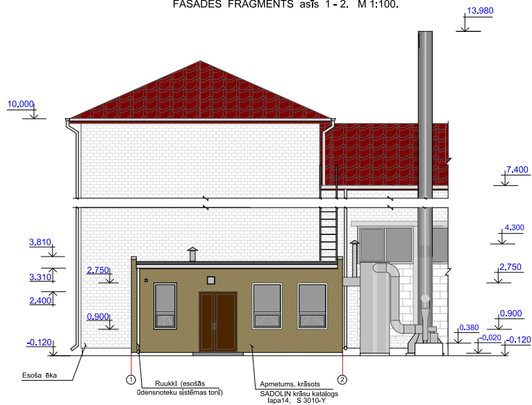
FASĀDES FRAGMENTS asis 1-2. M 1:100.
