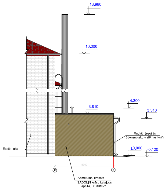
FASĀDES FRAGMENTS asis B - A. M 1:100.
